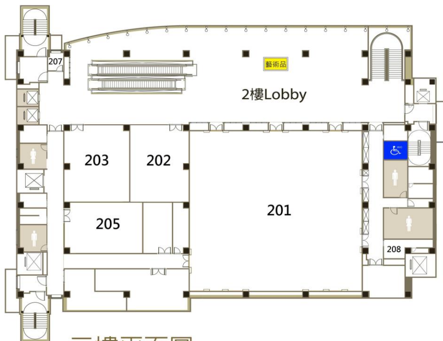
二樓平面圖
